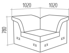
corner module модуль угловой
