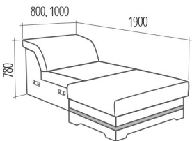
double module модуль двойной
