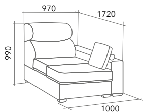
Секция шезлонг с подлокотником (правая, левая)
